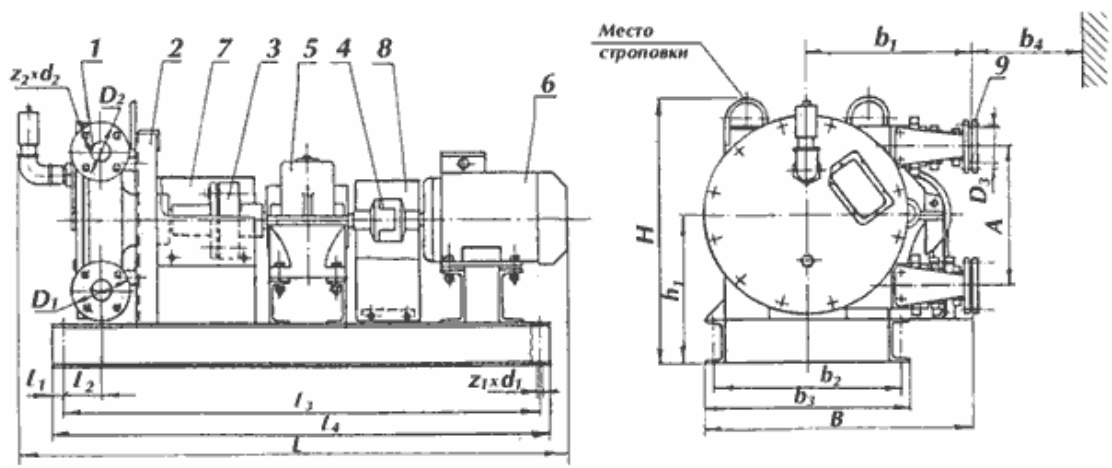
1.Насос 2.Рама. 3.Муфта упругая (для насоса НП-50 втулочно-пальцевая) 4.Муфта упругая (для насоса НП-50 втулочно-пальцевая) 5.Редуктор цилиндрический двухступенчатый 6.Электродвигатель асинхронный 7.Кожух 8.Кожух 9.Фланец ответный.
